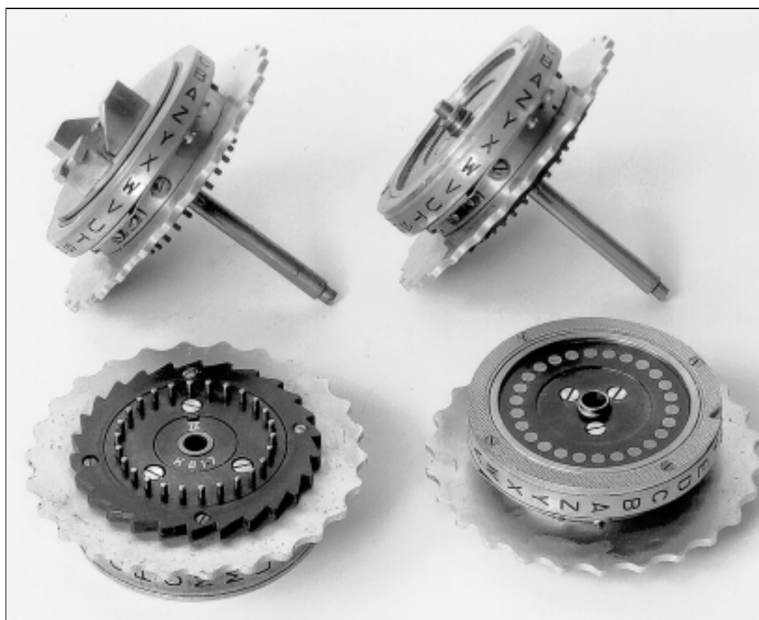
Walzen für die Enigma: Umkehrwalze mit Achse (oben links), Walze mit Klinkenrad und Federstiften (unten links), Walze mit Buchstabenring, Mitnahmekerbe und Kontaktflächen. (Bilder Günter Hüter)
